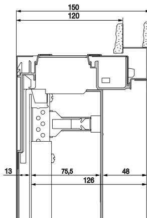
Rozvodnice s montážní deskou
